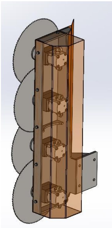
Modèle avec un moteur par scie
